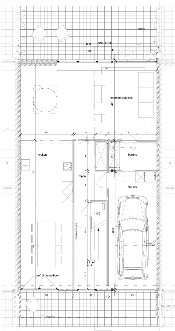
Gelijkvloers [1/100]
